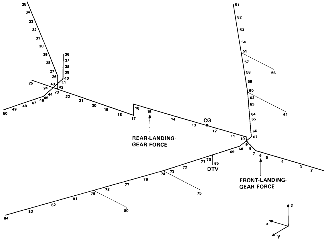
Fig. 3 B-52 NASTRAN model.
