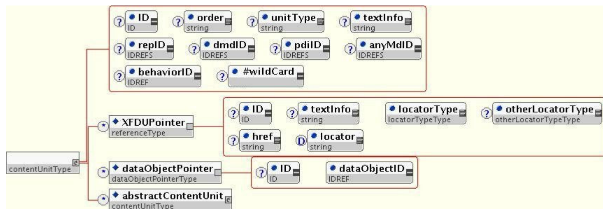
Figure 6-1: contentUnitType Schema Diagram
