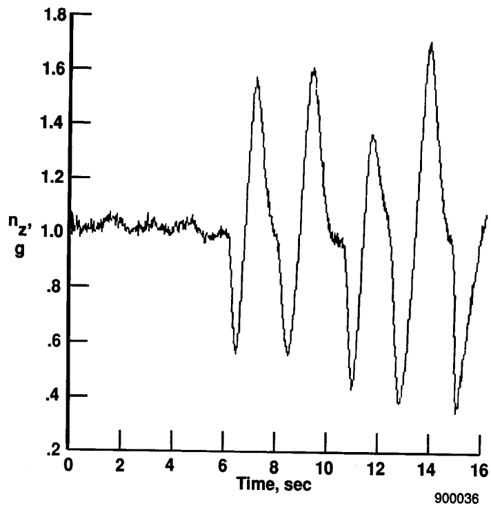
(d) Normal acceleration.
