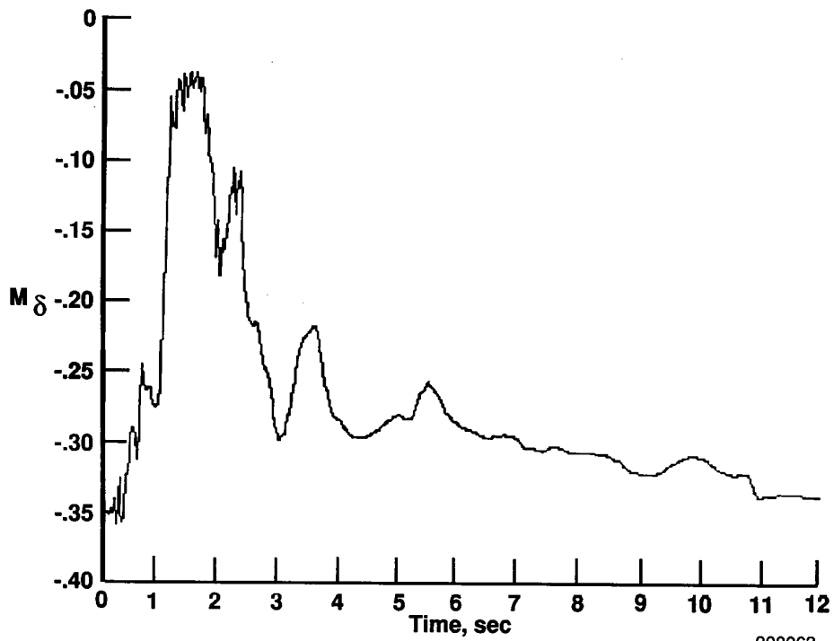
(d) M_{\delta} .
