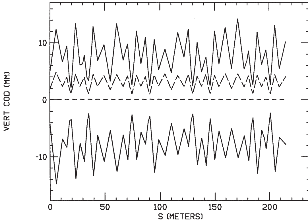
NSNS RING COD (MAX, MIN, RMS) Fig. 8a
