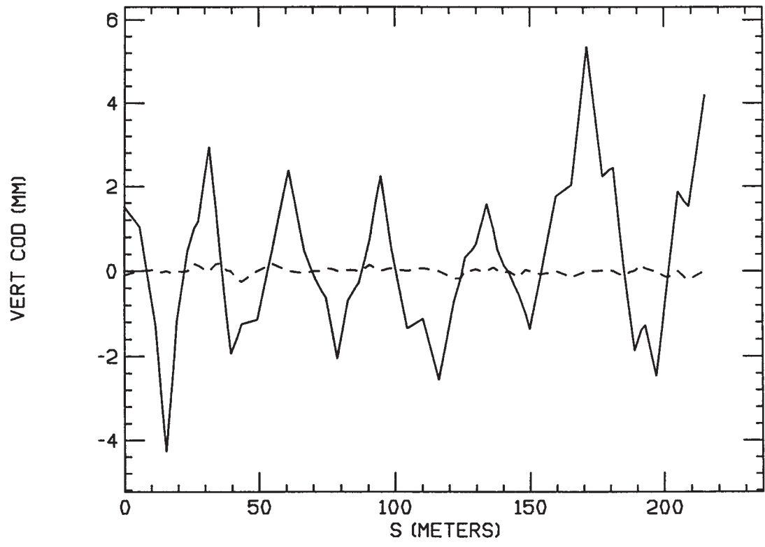
NSNS RING COD Fig. 7a
