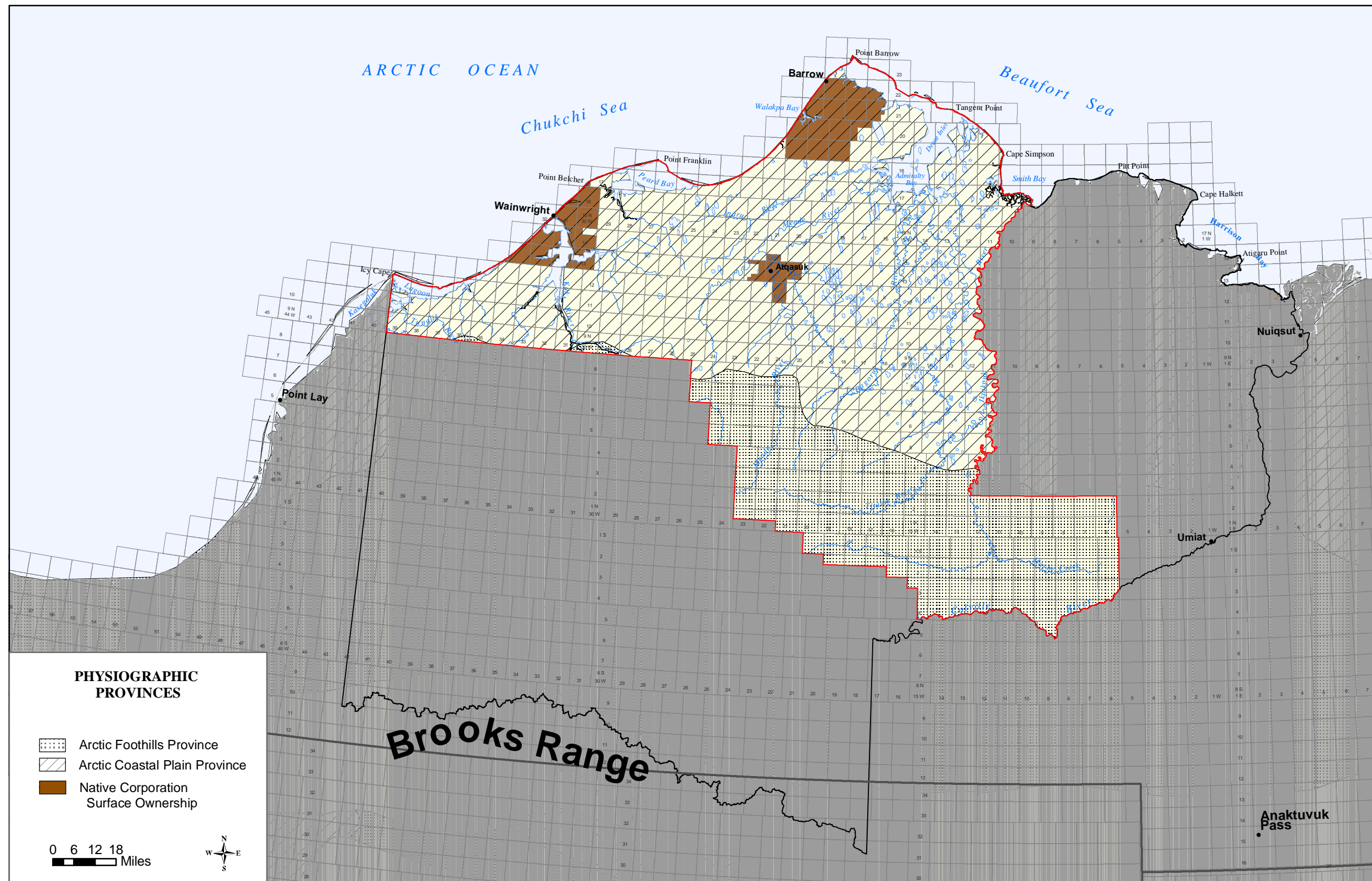
Source: Wahrhaftig, 1965 Map 28. NW NPR-A Physiographic Provinces
