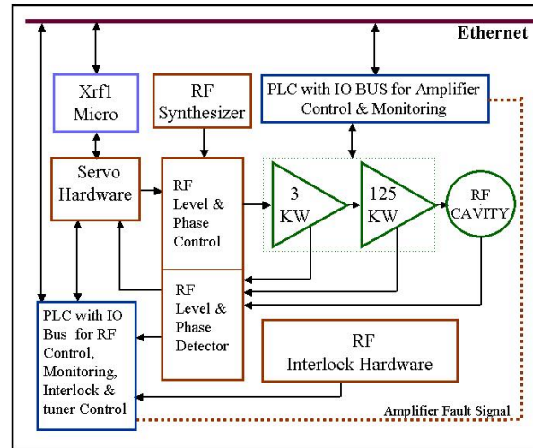
Fig. 1 X-ray RF1 System
