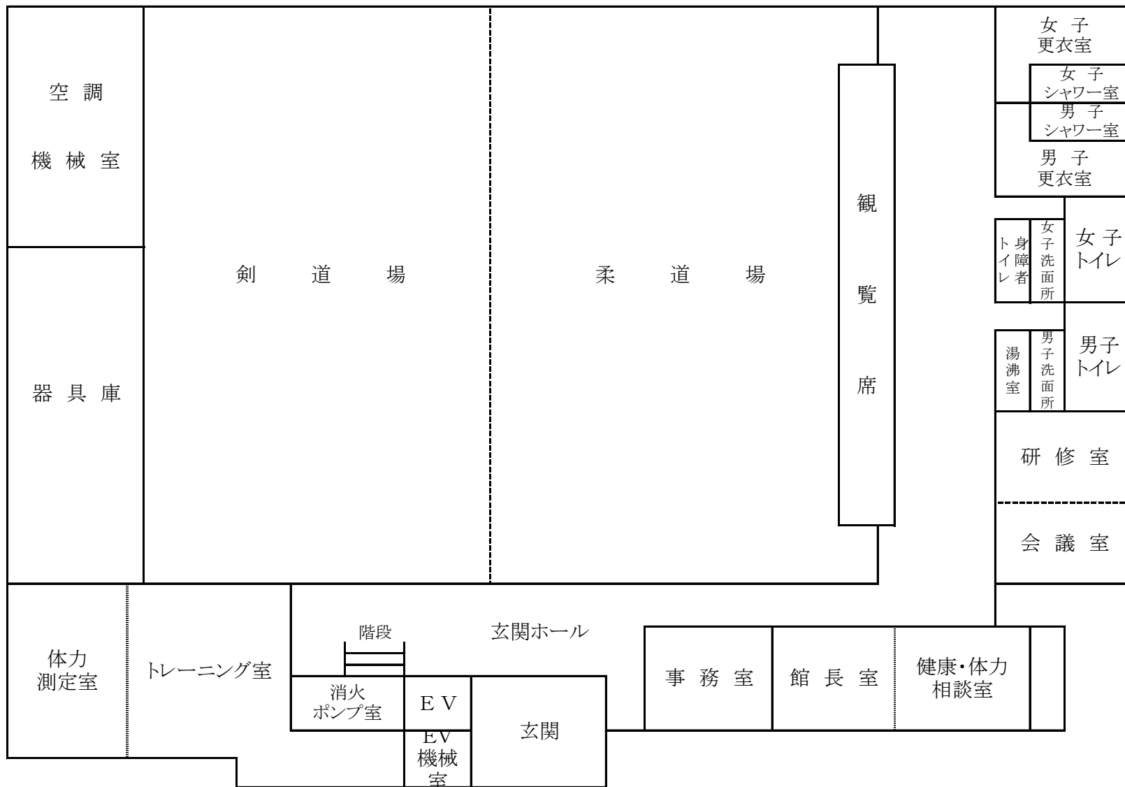
1 FL 平面図
