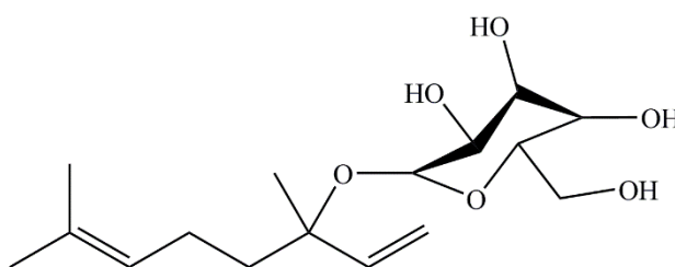
linalol – glikozid
