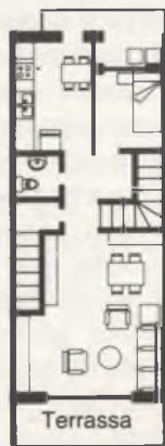
PLANTA PIS 1r.
