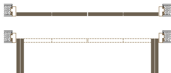
Схема открывания складной двери из четырех полотен.
