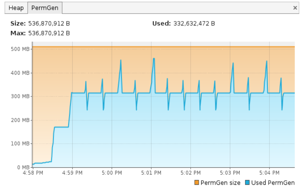
Drools 6 - 15 loops
