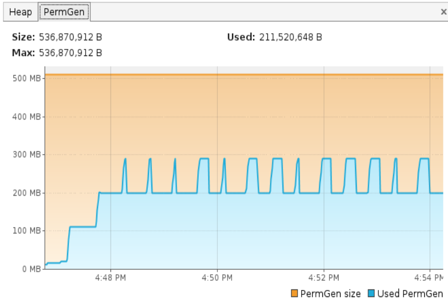
Drools 5 - 15 loops
