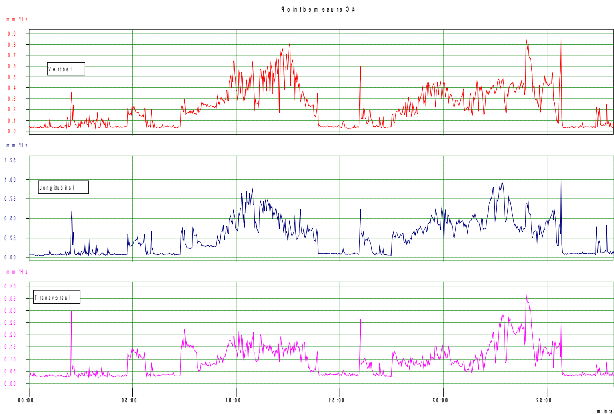
Palplanches 1 – Capteur C4
