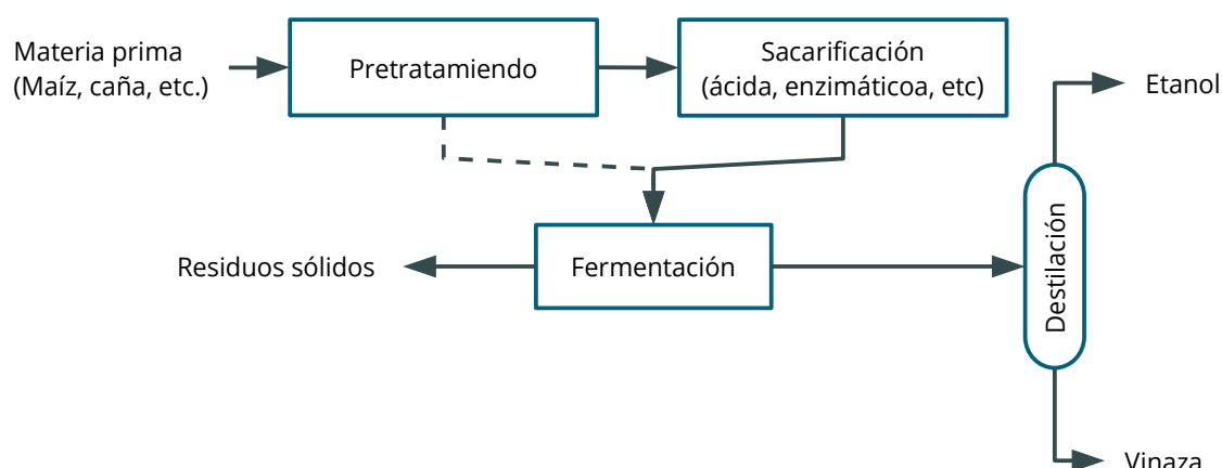
Figura 1.4: Esquema simplificado de producción de bioetanol [12][15]. La línea sólida representa el proceso convencional, mientras la línea rayada implica un tratamiento de hidrólisis y fermentación simultáneo.
