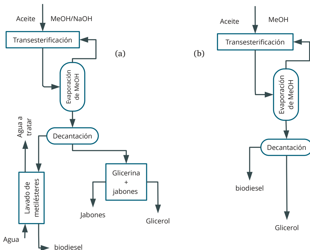
Figura 1.3: Esquema simplificado de producción de biodiesel de metanol. (a) Proceso catalítico. (b) Proceso supercrítico.[5]
