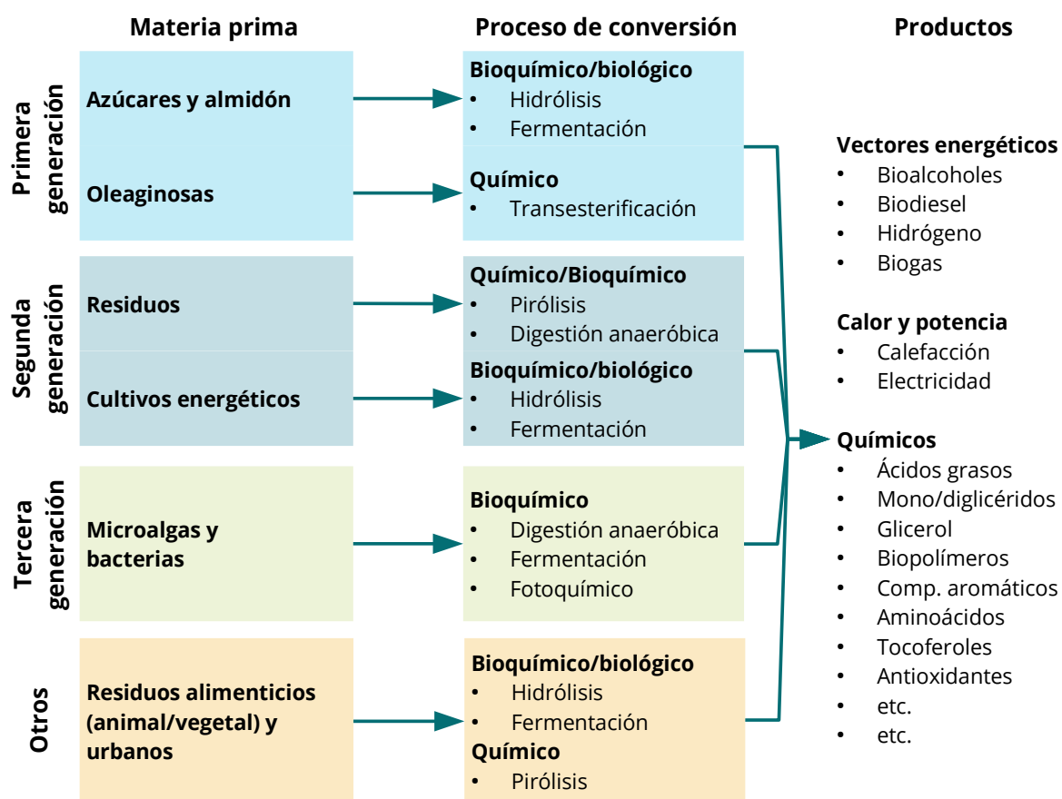
Figura 1.2: Resumen de las principales distintas materias primas de biomasa, los procesos de conversión y productos finales asociados a biorrefinerías.
