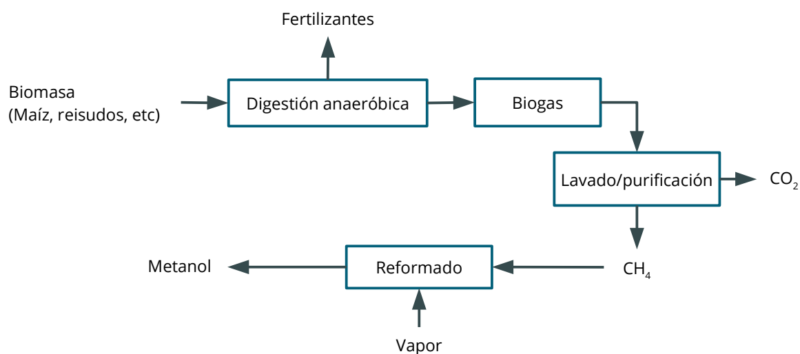
Figura 1.6: Esquema simplificado de producción de biometano por digestión anaeróbica y/o biometanol por posterior reformado[14].
