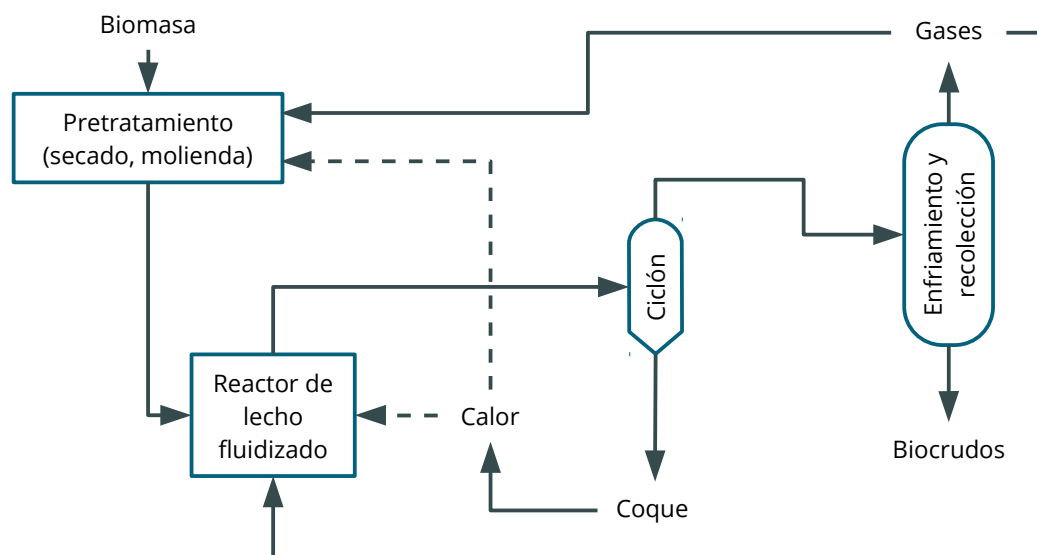
Figura 1.5: Esquema del proceso de pirólisis rápida sobre lecho fluidizado para obtener biocrudos[14].
