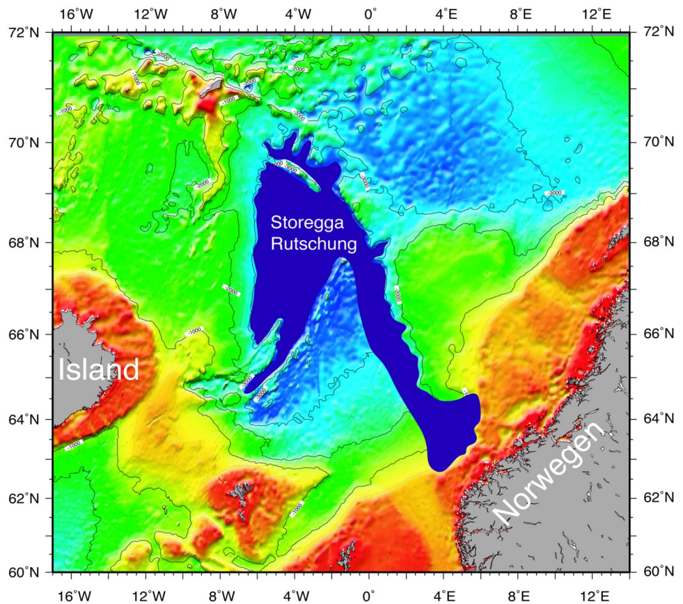
Abb. 10: Storegga Rutschung als Beispiel für Hanginstabilitäten, die durch Gashydratzersetzung ausgelöst werden können. Die Abrissnische liegt am norwegischen Kontinentalhang in einer Wassertiefe nahe der Phasengrenze der Gashydrate. Die Rutschmasse verteilt sich über das tiefe Norwegen Becken entlang der Bodenmorphologie. Die Storegga Rutschung ist mit über 5.600 km 3 Gesamtvolumen eine der größten bekannten submarinen Rutschungen.
