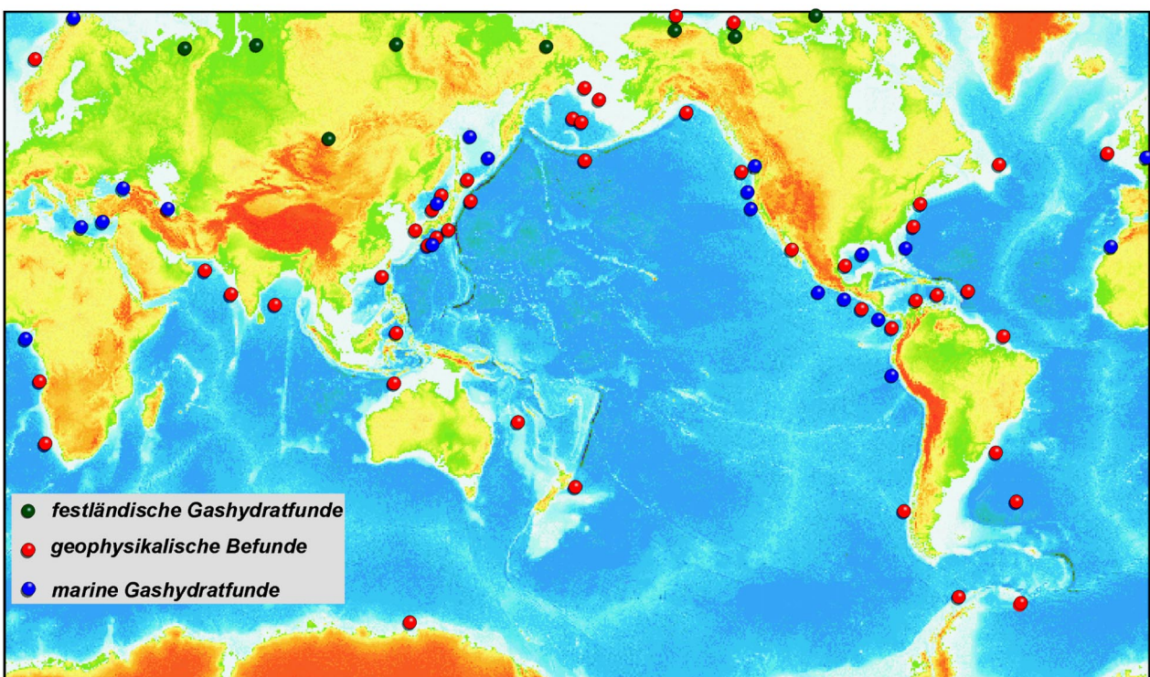
Abb. 4: Weltweite Verbreitung der Gashydratvorkommen im Bereich der Dauerfrostböden an Land (grüne Punkte) und entlang der Kontinentalränder im Ozean. Die überwiegende Zahl der Vorkommen im marinen Bereich wurden
