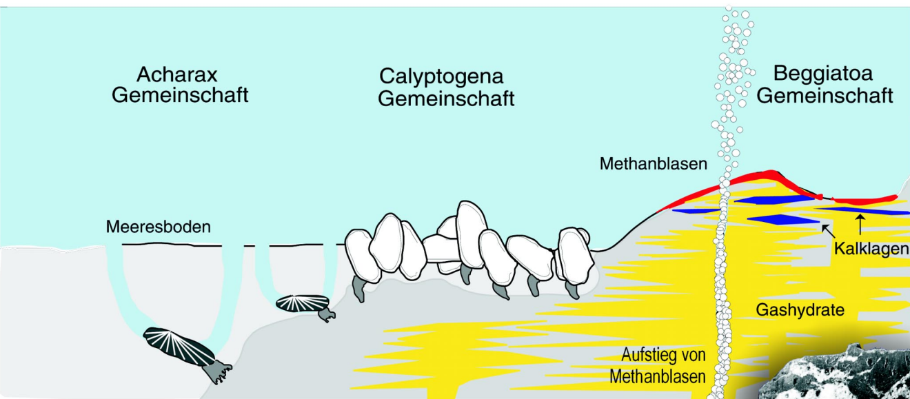
Abb. 8: Oben: Gashydrate am Meeresboden und die Verteilung ihrer typischen Faunengemeinschaften aus Muscheln und Bakterien. Die Gashydrate bilden sich, wenn aufsteigende Methanblasen aus tieferen Sedimentschichten mit Wasser in Kontakt kommen. Gashydrate bilden ein fast unerschöpfliches Substrat für den mikrobiellen Umsatz von Methan im oberflächennahen Sediment. Hierbei entstehen große Mengen an Schwefelwasserstoff, die wiederum als Energielieferant für die hier dargestellten drei chemoautotrophen Gemeinschaften dienen. Dabei kommt es auch zu einer Ausfällung von Kalken, die häufig zusammen mit Gashydratlagen vorkommen. Rechts: Gashydratprobe vom Meeresboden. Das Bild zeigt ein senkrecht zur Schichtung durchsägtes Handstück mit unterschiedlich dicken Lagen von weißem Gashydrat in dunklem Sediment. Das Sedimentgefüge wurde durch die Gashydratbildung völlig verändert. Foto: GEOMAR
