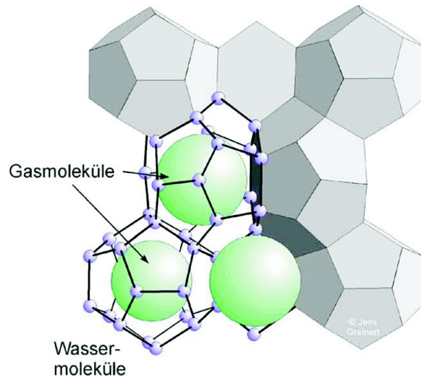
Abb. 2: Die Gashydratstruktur (hier Struktur I) besteht aus Wasserkäfigen, die Gasmoleküle einschließen. Die Wassermoleküle bilden in charakteristischer Weise die Eckpunkte der Käfige in denen je ein Gasmolekül (Methan, Kohlendioxid, Schwefelwasserstoff oder andere Gase) Platz findet. In der Natur treten mehrere Käfigtypen mit unterschiedlichen Volumina auf, so dass unterschiedliche Gasmoleküle eingebaut werden und zur Stabilisierung der Gashydratstruktur beitragen. Abb. aus Suess et al., 1999.
