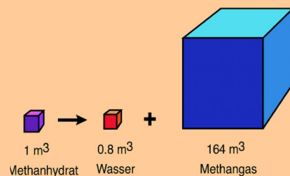
Abb. 7: Vergleich von einer Volumeneinheit (1 m 3 ) Methanhydrat und dem darin gespeicherten 164-fachen Volumen an Methangas.
