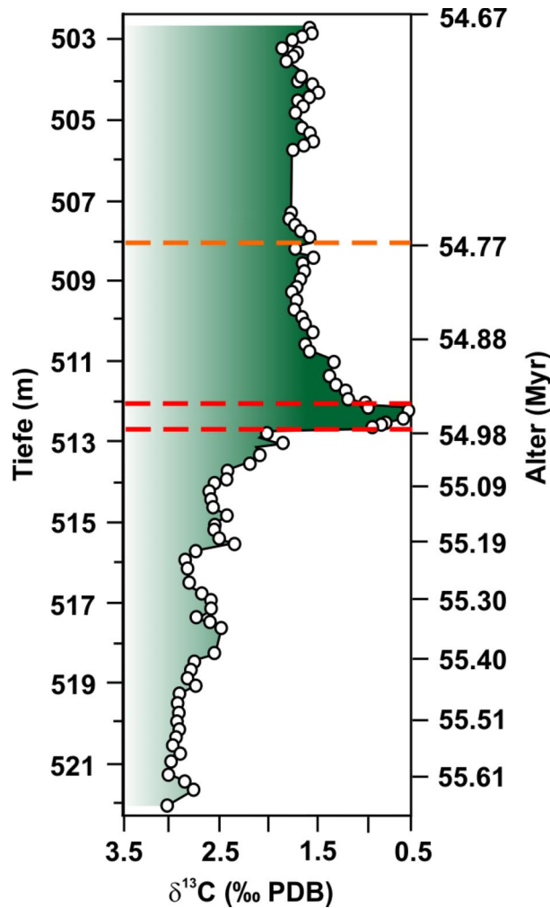
Abb. 11: Verlauf des Kohlenstoffisotopensignals aus Foraminiferenschalen über das spät-Paläozäne Klimaoptimum, etwa 55 Mill. Jahren vor heute. Die starke Zunahme des leichten 12 C wird auf die Zumischung von Kohlenstoff aus Methanhydrat in die globale Umwelt zurückgeführt. Berechnungen zufolge ist ein Methan-Puls von ca. 1 Gigatonne Kohlenstoff aus Gashydrat über 20.000 Jahre notwendig (gestrichelte rote Linien), um ein solch globales Signal zu verursachen. Ein Einschnitt der Faunenvergesellschaftungen im Ozean und an Land gehen mit diesem Puls in der Kohlenstoffisotopie einher, der langsam über einen Zeitraum von 200.000 Jahren wieder abklingt (obere gestrichelte rote Linie).
