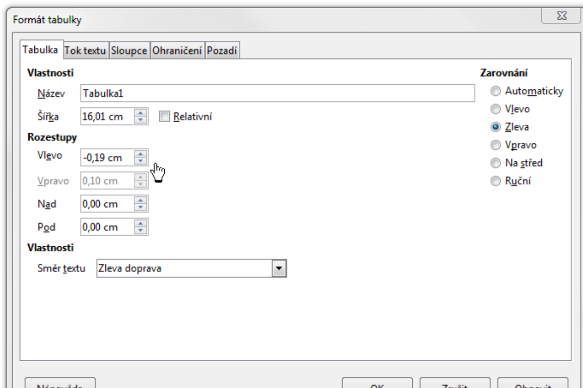
1. Ilustrace: LO 4.4.2
