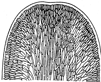
⑨ Flechtgewebe
