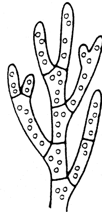
⑦ siphonocladal
