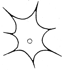
② rhizopodial
