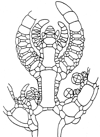
⑩ Gewebe-Thallus
