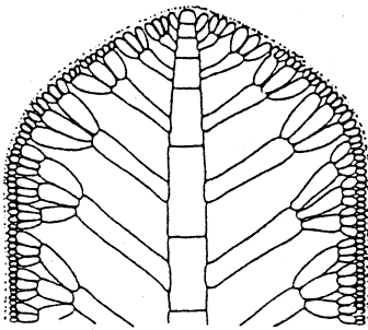
⑧ Zentralfaden-Typ
